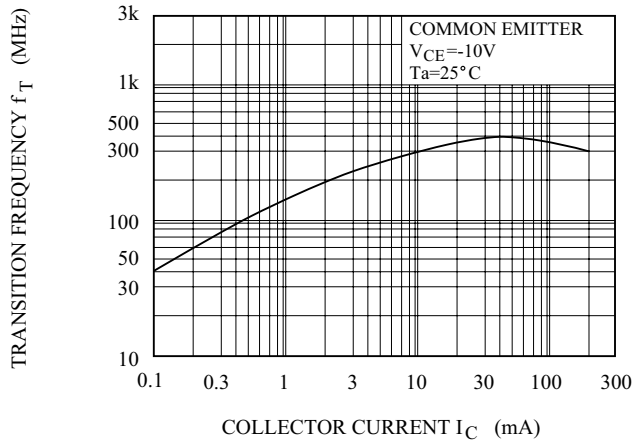
f_T - I_C
